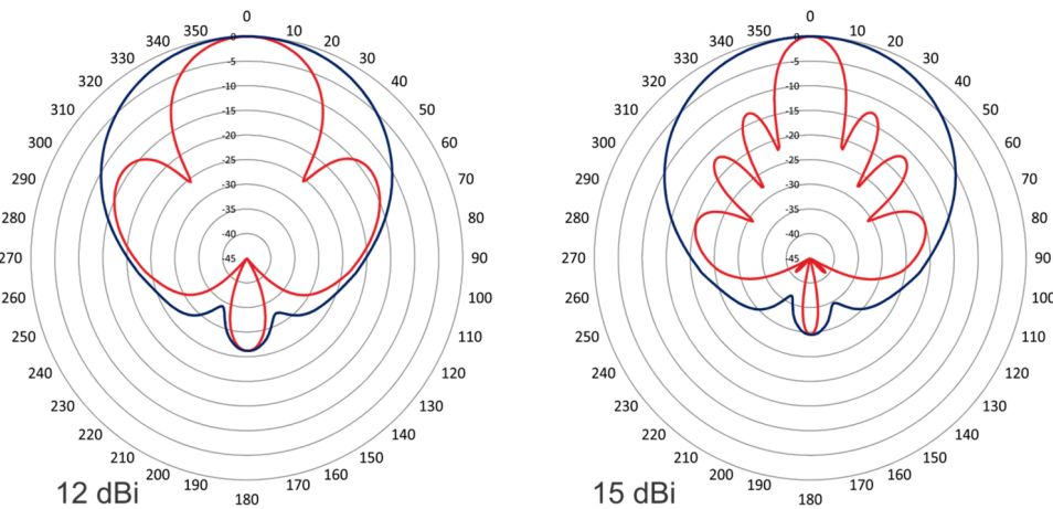
Diagramas de referência aplicáveis aos modelos de 12 dBi e 15 dBi.
